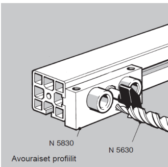
Kuvaus: Poraohjain 13,5 mm perusosa. Avouraisille profiileille
