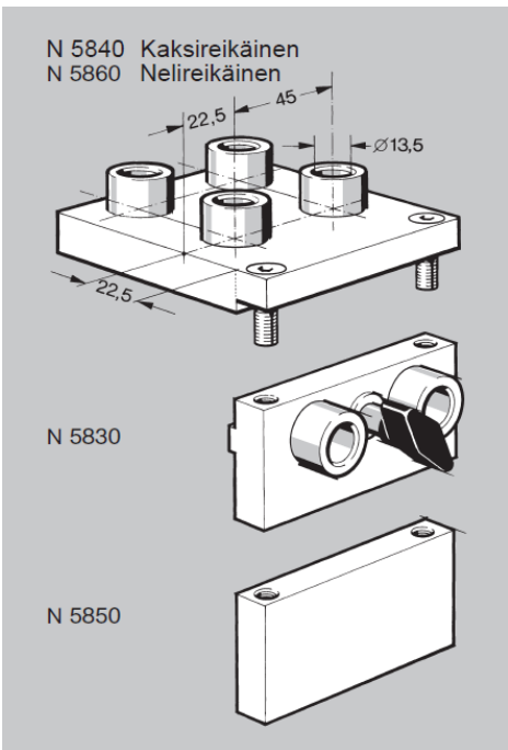
Kuvaus: Poraohjain 13,5 mm perusosa. Avouraisille profiileille
